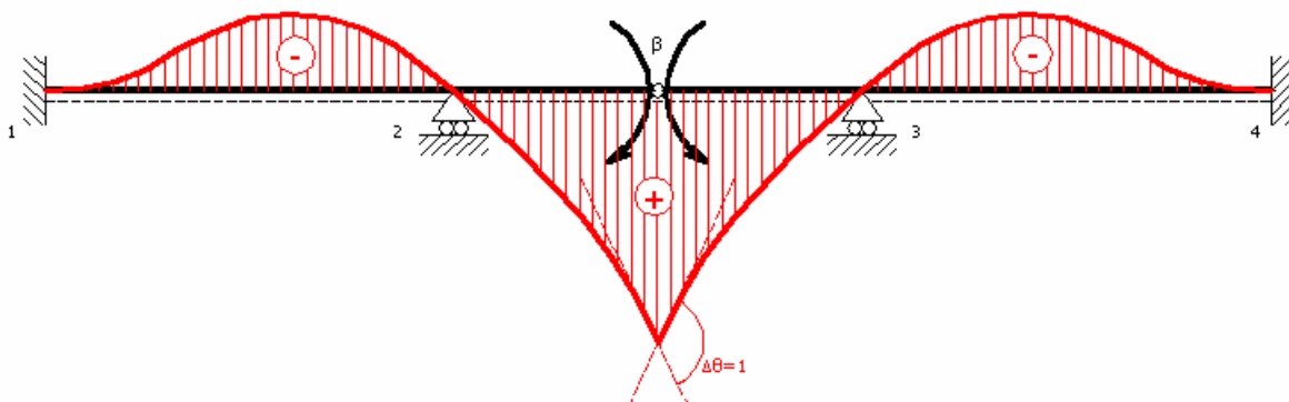
Γραμμή Επιρροής M_\beta
