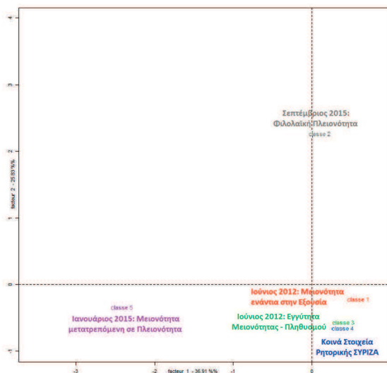
Γράφημα 2 Προβολή στο παραγοντικό διάγραμμα (1,2) της Παραγοντικής Ανάλυσης Αντιστοιχιών, των πέντε κλάσεων λεκτικού υλικού των προεκλογικών ομιλιών του Α. Τσίπρα (Μάιος-Ιούνιος 2012, Ιανουάριος 2015 και Σεπτέμβριος 2015)
