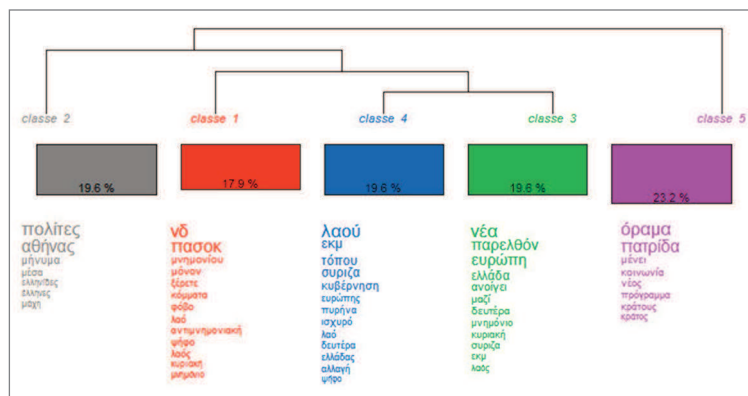
Γράφημα 1 Δενδρόγραμμα ιεραρχικής ταξινόμησης λεκτικού υλικού των κεντρικών προεκλογικών ομιλιών του Α. Τσίπρα (Μάιος 2012-Σεπτέμβριος 2015)
