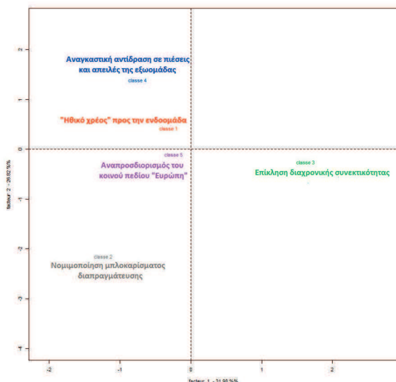
Γράφημα 4 Προβολή στο παραγοντικό διάγραμμα (1,2) της Παραγοντικής Ανάλυσης Αντιστοιχιών των πέντε κλάσεων ηλεκτικού υλικού του διαγγέληματος και της ομιλίας του Α. Τσίπρα σχετικά με τη διενέργεια Δημοψηφίσματος
