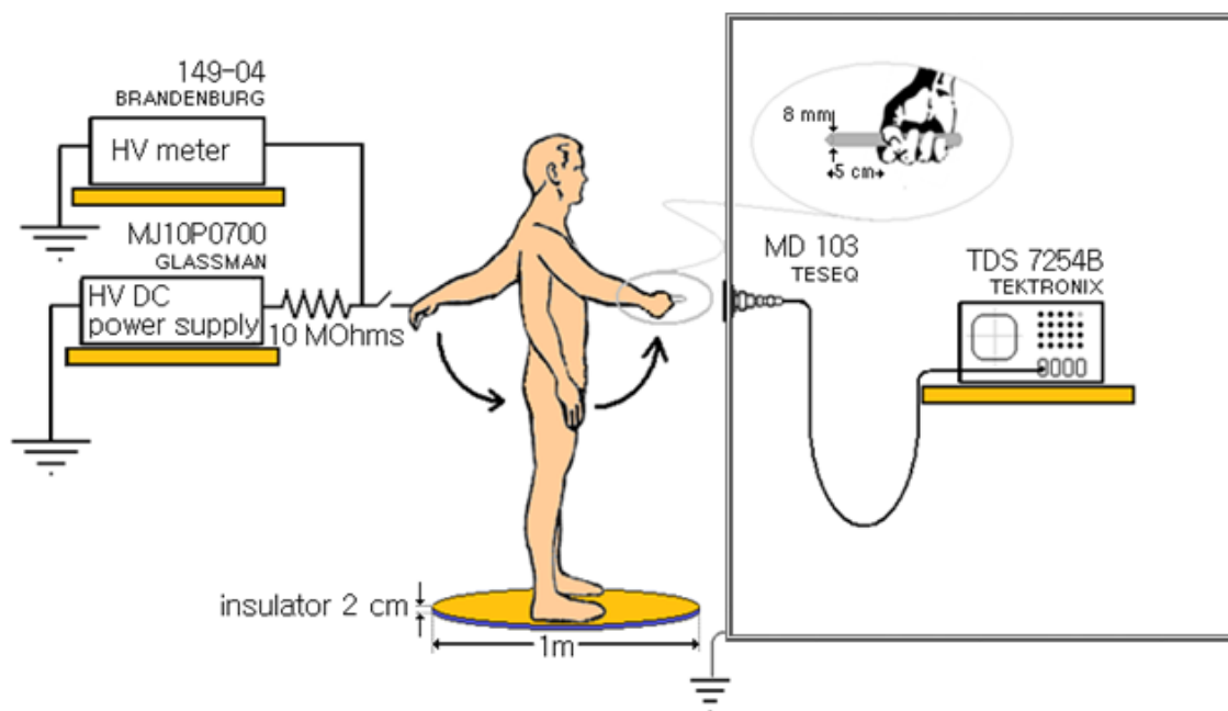
Σχήμα 1. Πειραματική διάταξη
