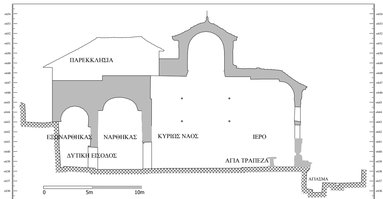
Σχήμα 3. Καταμήκος τομή καθολικού
