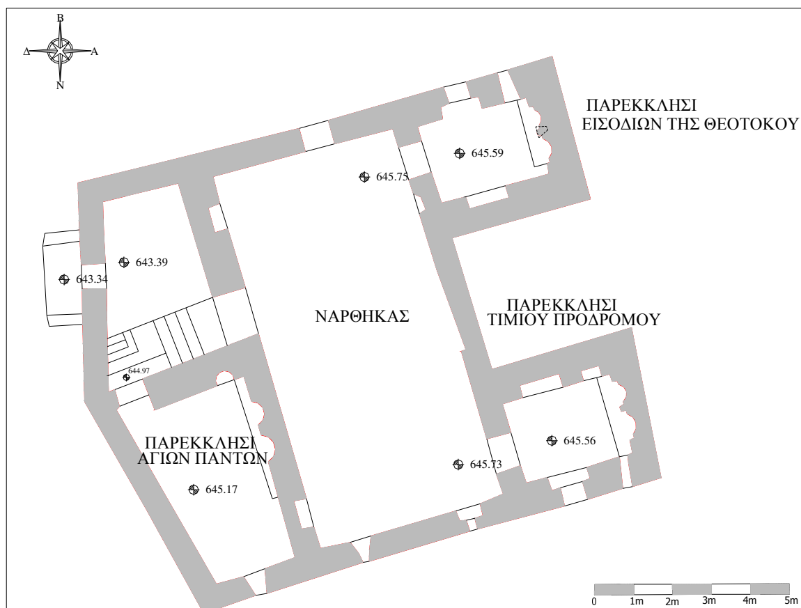
Σχήμα 2. Κάτοψη παρεκκλησίων
