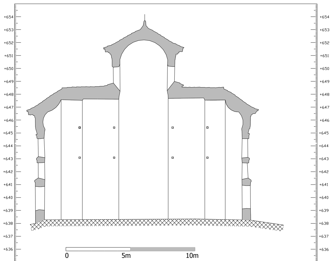
Σχήμα 4. Εγκάρσια τομή στο χώρο του κυρίως ναού
