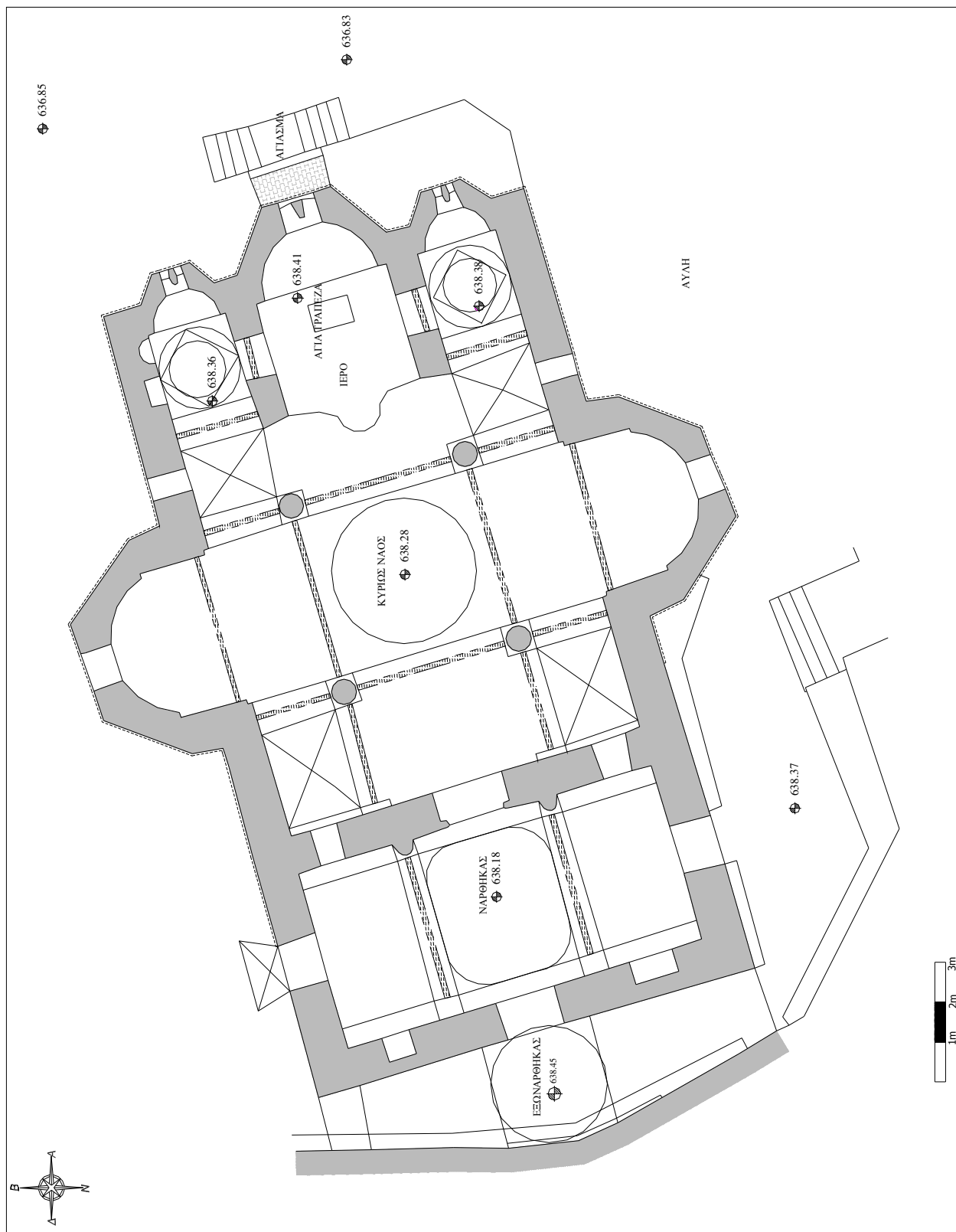
Σχήμα 1 Οριζόντια τομή καθολικού
