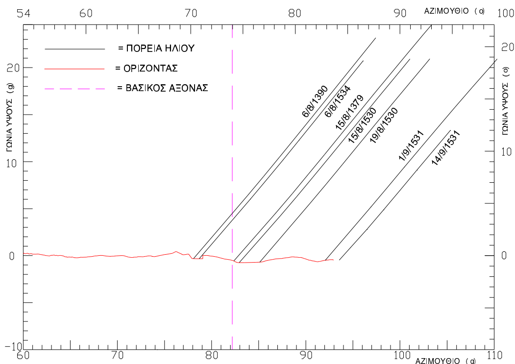
Σχήμα 6. Σύνθετο διάγραμμα ορίζοντα, βασικού άξονα και πορειών ήλιου.
