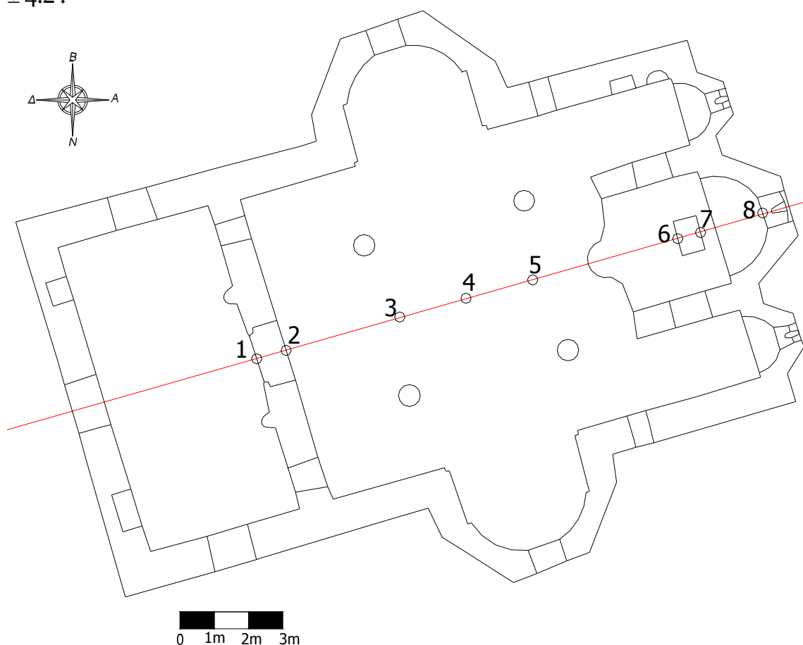
Σχήμα 5. Βασικός κατά μήκος άξονας καθολικού
